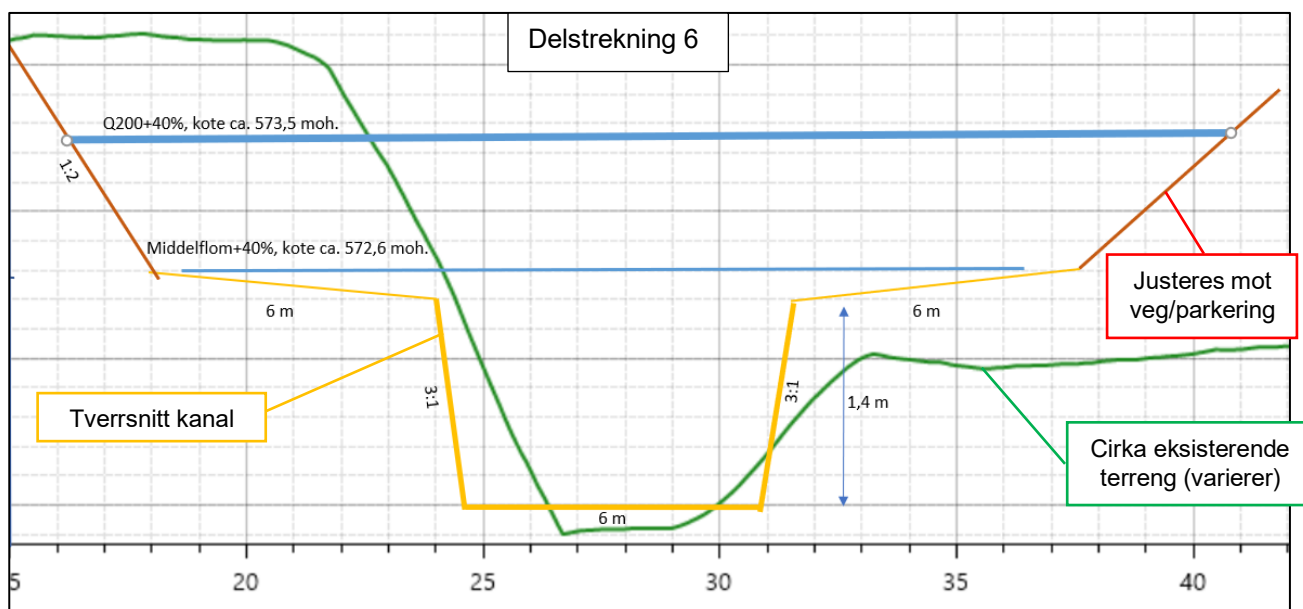
Figur 11: Prinsipp for tverrprofil av kanalen for delstrekning 6 (nedstrøms Bjorlivegen), vist med 6 meter brede traseer for skiløyper/gangveg på hver side. Kanalen avsluttes til høyre i figuren mot vegfyllingen/parkeringsplassen som er planlagt langs nordsiden av kanalen
