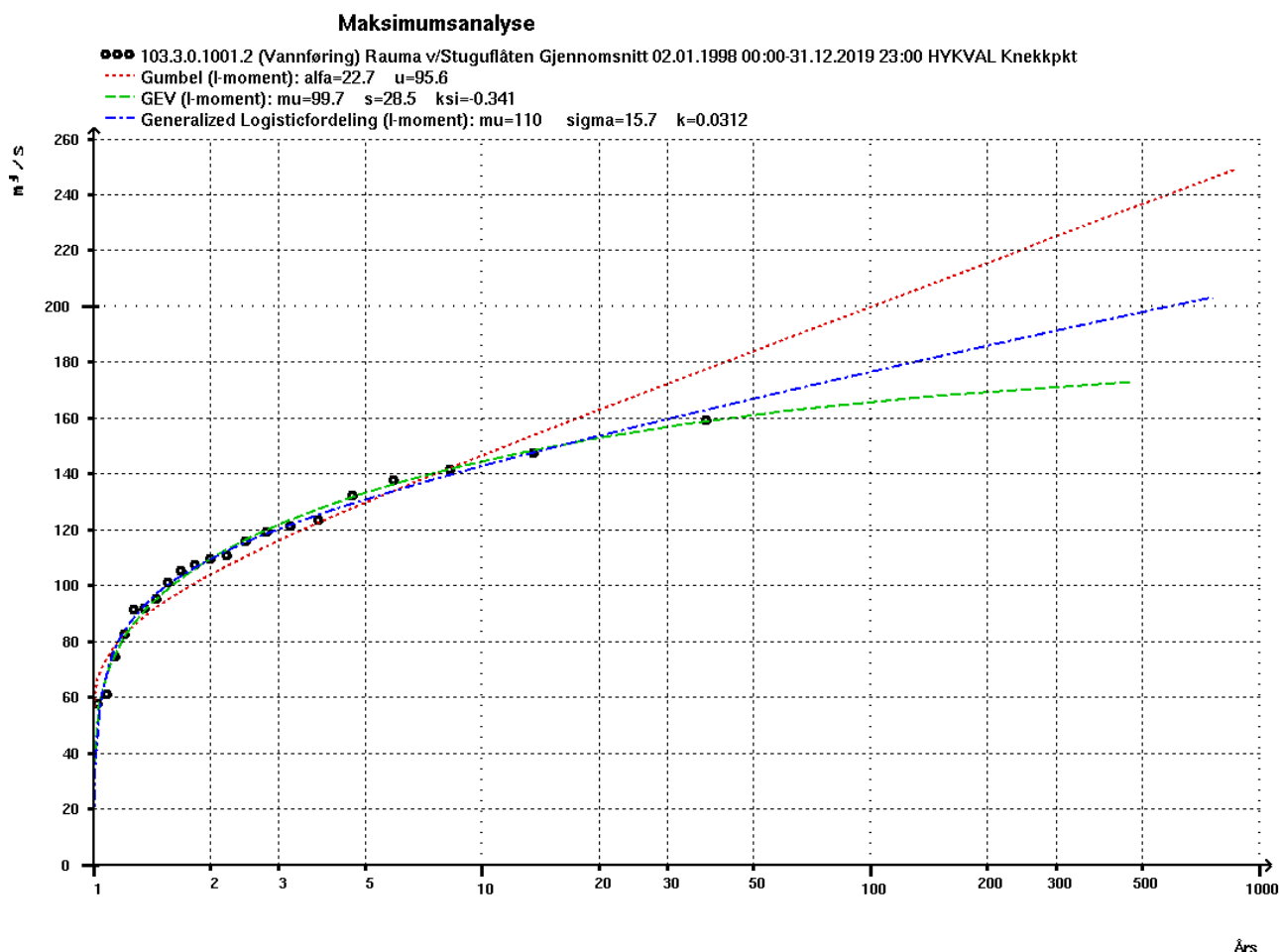
Figur 4: Flomfrekvensanalyse for målestasjonen ved Stuguflåten.
