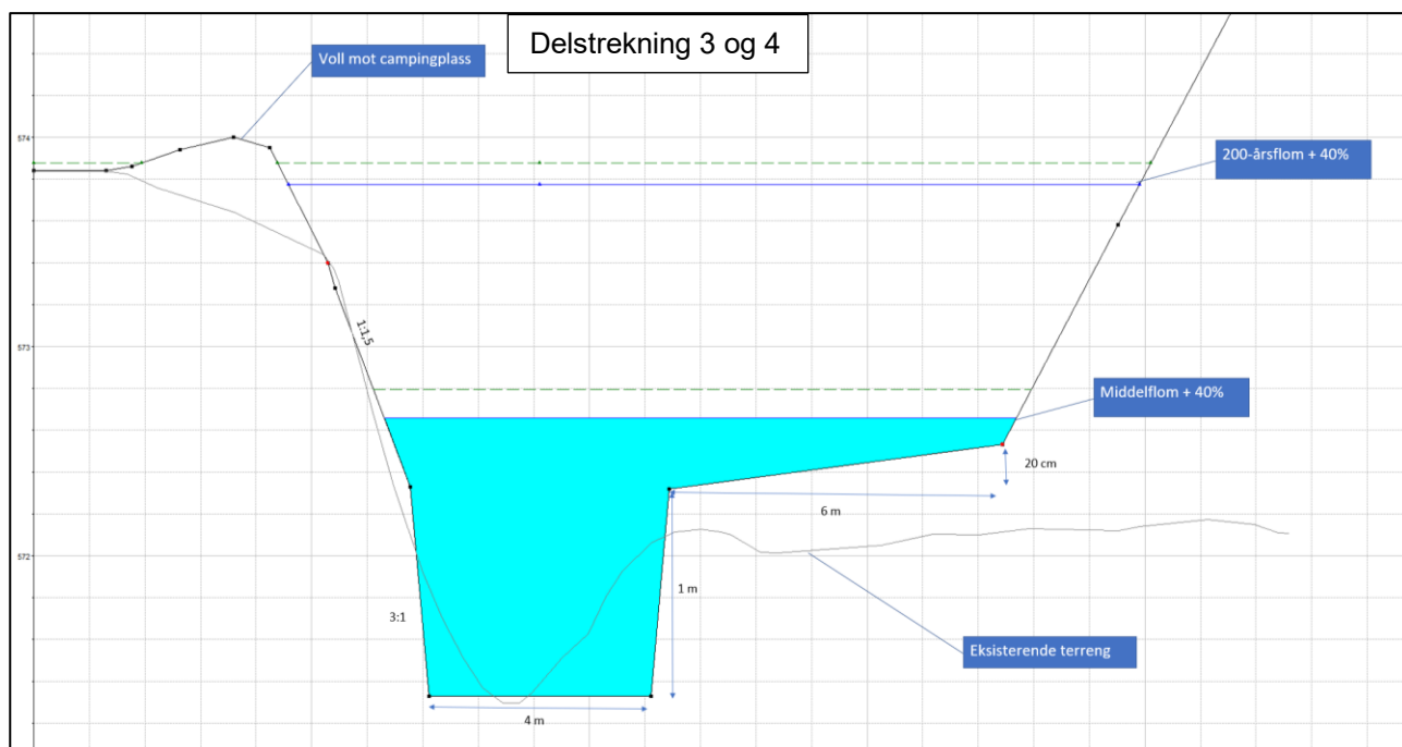
Figur 10: Prinsipp for tverrprofil av kanal for delstrekningene 3 og 4, sett i nedstrøms retning.
