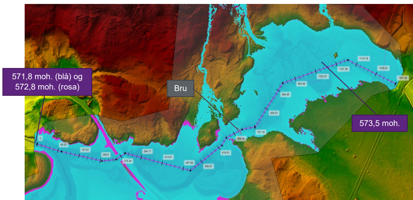
Figur 7: Resultat av to flomsimuleringen ved to ulike grensebetingelser i Rauma. Rosa farge viser flomsone for vannstand lik 572,8 moh. i Rauma, mens blått viser flomsone for vannstand lik 571,8 moh. i Rauma. Vannstanden i myrområdet blir tilnærmet lik i begge simuleringer.
