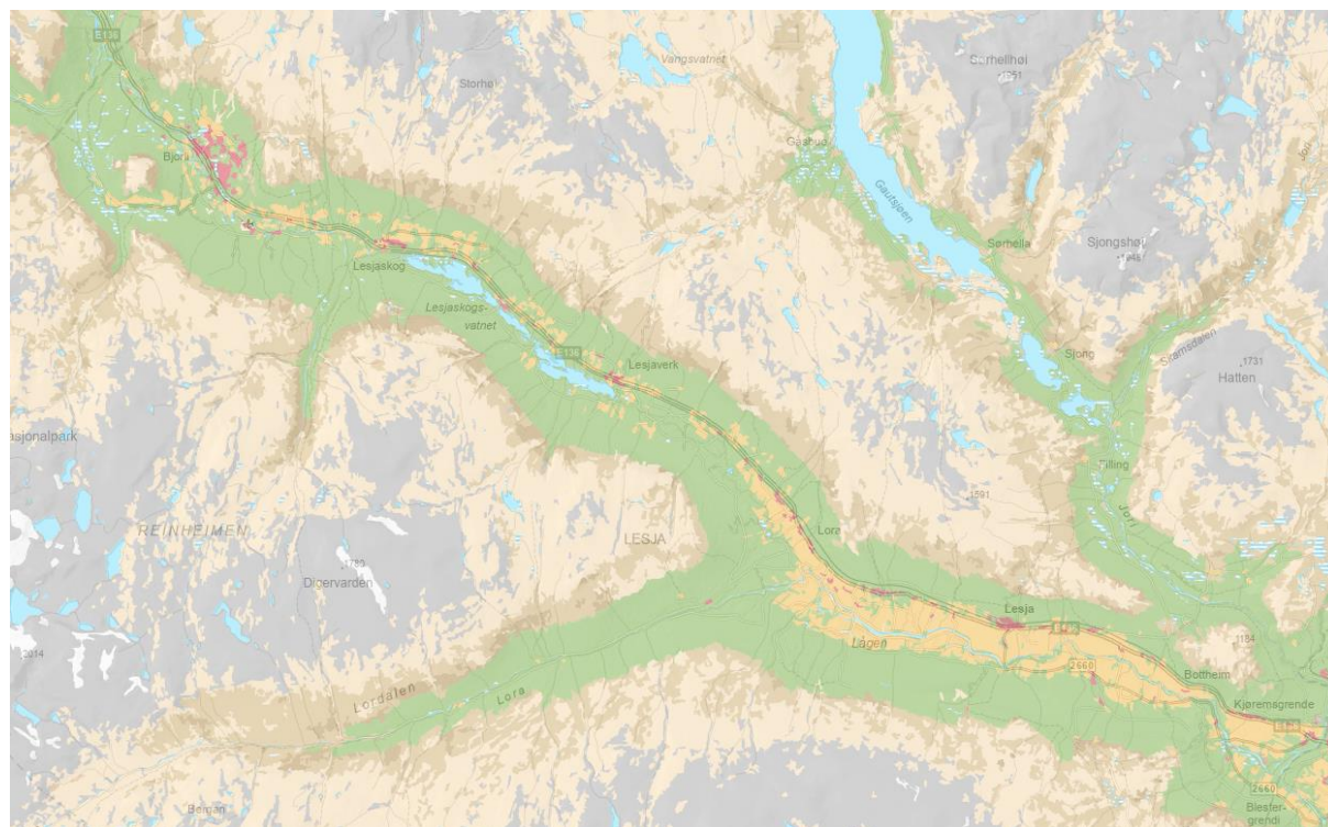
Figur 2: Visar utsnitt av Lesja kommune med framvisning av arealtypar i farger.
